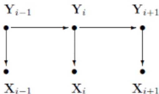
Figura 8. Modelo gráfico de un HMM.
