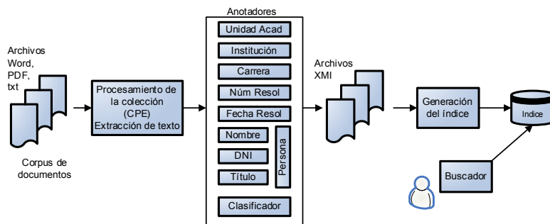
Fig.1. Arquitectura del sistema
