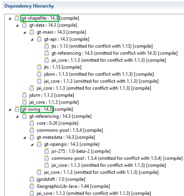
Figura 2. Dependencias directas y transitivas requeridas por el programa Quickstart de GeoTools.
